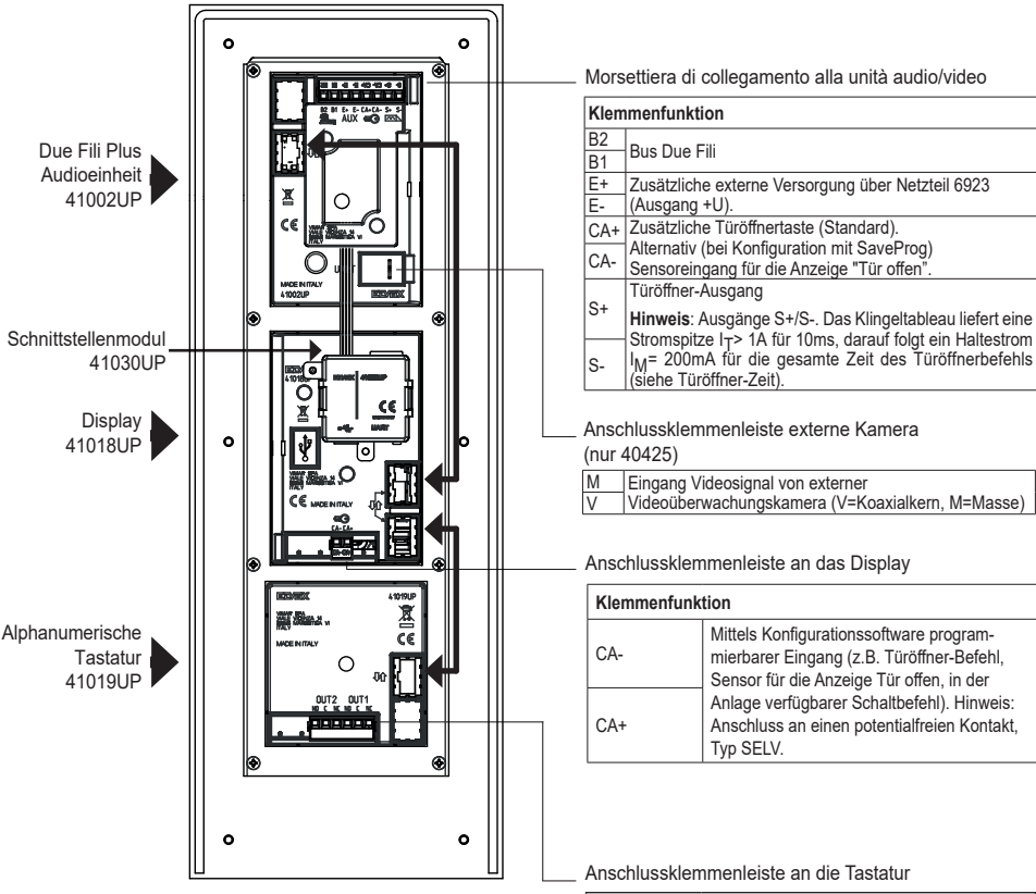
Rückansicht des Audio-Klingeltableaus 40425
