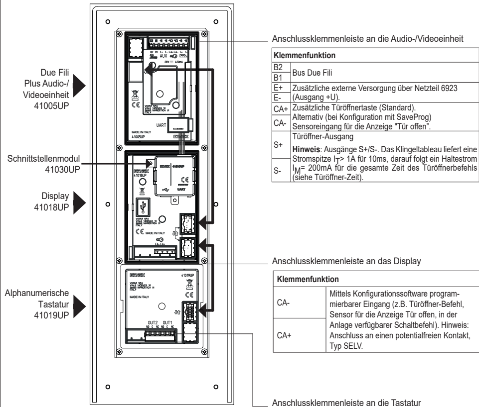
Rückansicht des Audio-/Video--Klingeltableaus 40405
