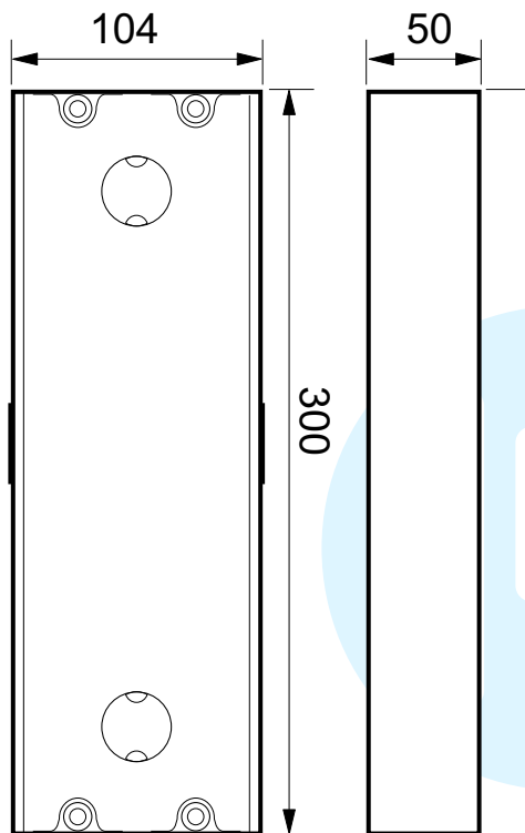
Inbouwdoos
